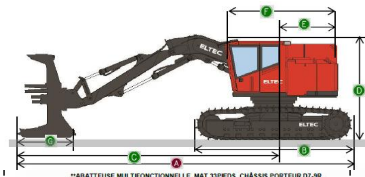
**ABATTEUSE MULTIFONCTIONNELLE, MAT 33PIEDS, CHÂSSIS PORTEUR D7-9R
